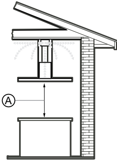
Instalación recirculante
